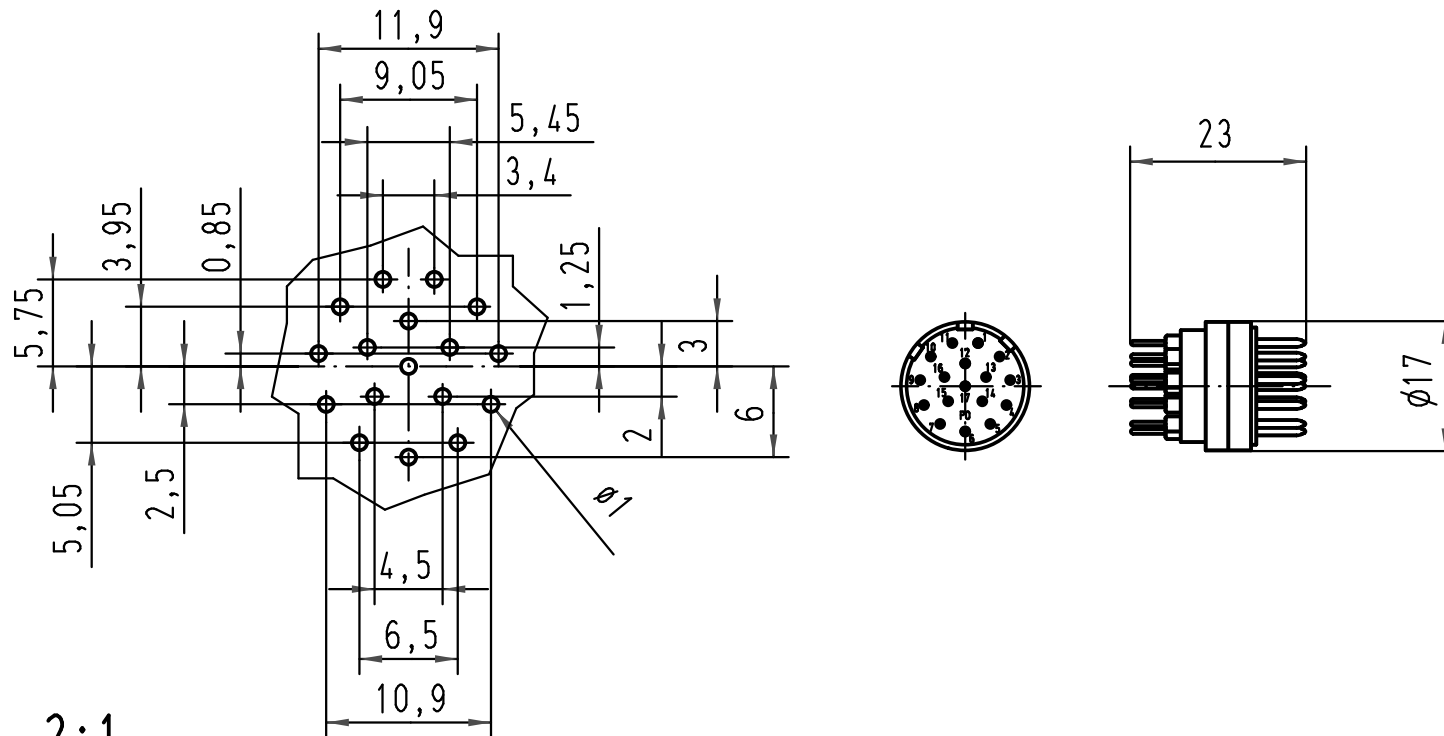
Lochbild/pinhole pattern
