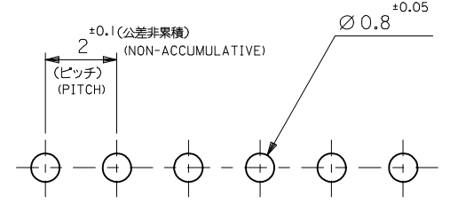
基板取付穴推奨寸法
