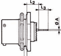
Receptacle type 7
