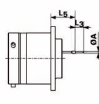
Receptacle type 2
