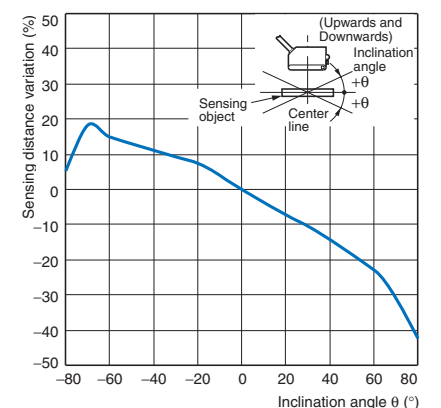
E3ZM-LS□4H(LS□9H)
