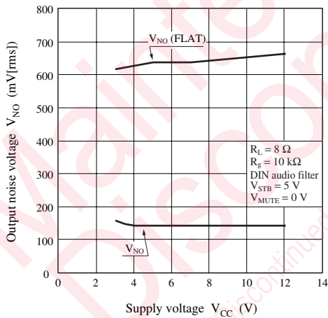
V_{\text{NO}} — V_{\text{CC}}
