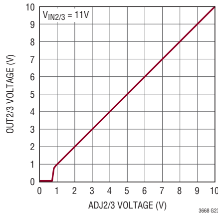
LDOs: Tracking
