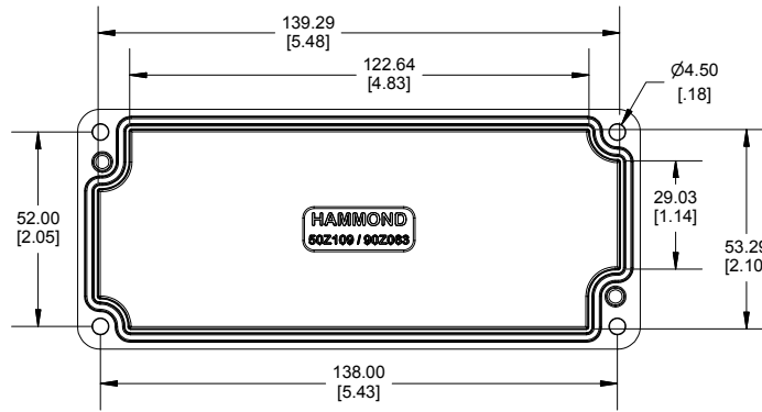
INSIDE LID
