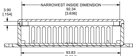
SECTION D-D
