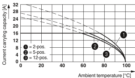
Type: MSTBT 2,5 HC/...-ST with MSTBVA 2,5 HC/...G
