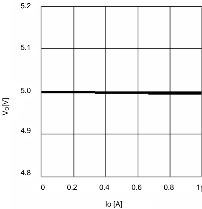
Fig.25 I_O - V_O
