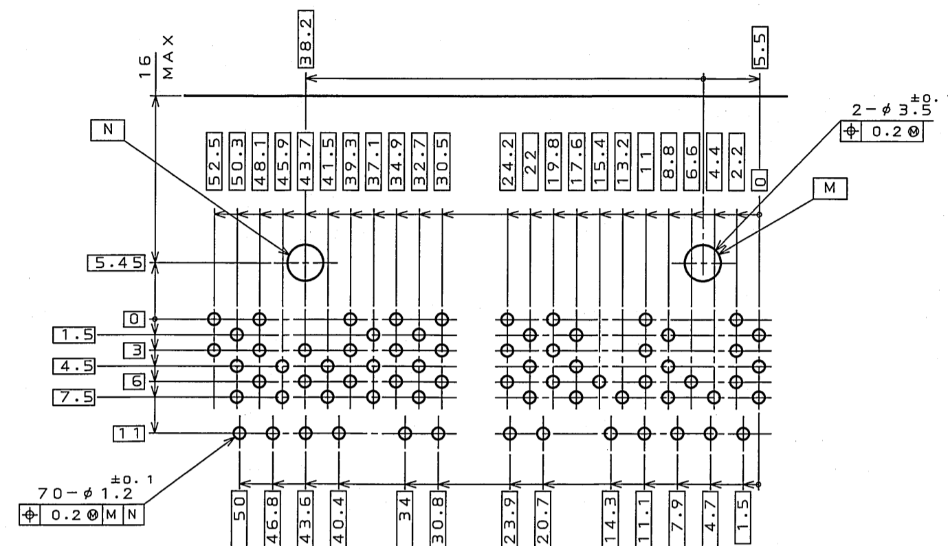
P.C.B. HOLE PATTERNS (REF.) 基板取付寸法(参考)
