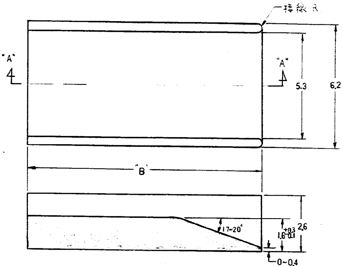
断面 "A-A"
